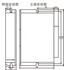
采用侧面安装，散热效果较好
