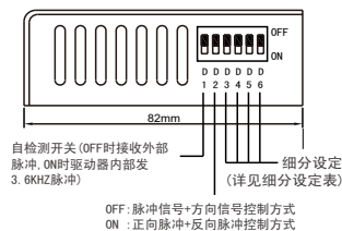
DIP开关功能设定示意图
